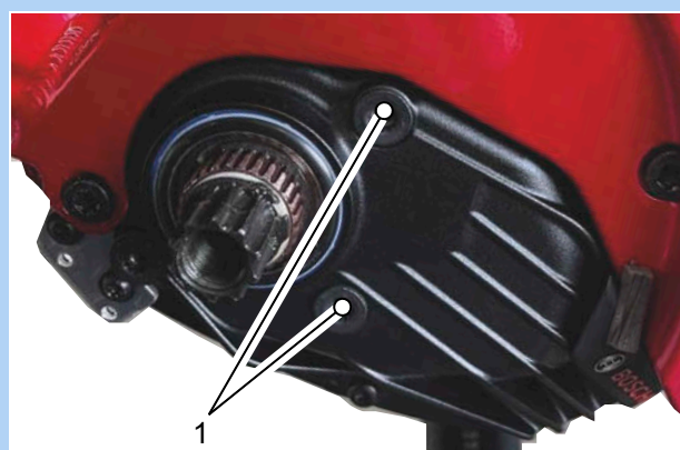
Figura 119: Ubicazione delle viti di fissaggio (1)
