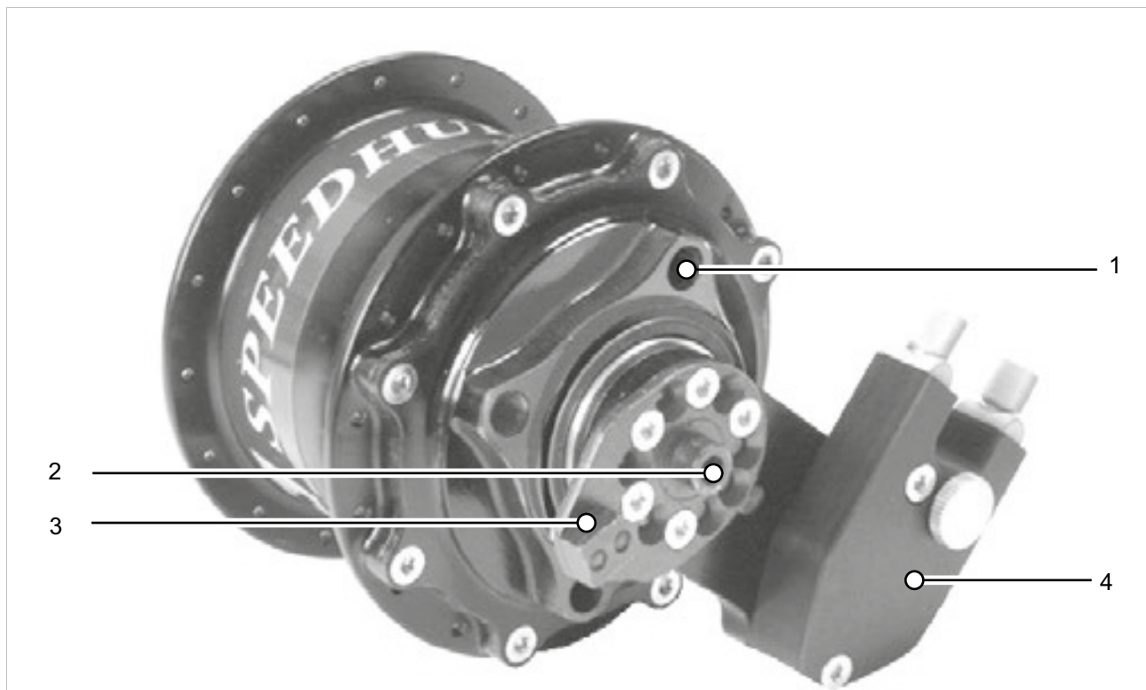
Figura 94: Dati tecnici e funzioni ROHLOFF, Speedhub 500/14 CC DB OEM, black, 32 holes, con coperchio freno a disco (1), asse a bloccaggio rapido (2), piastra di lavoro CC OEM (3) e comando esterno del cambio (4)
