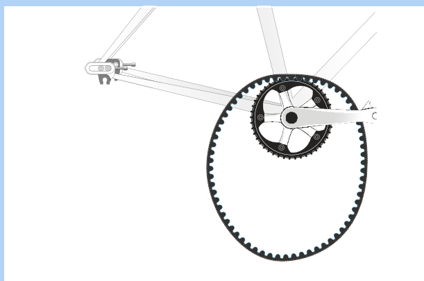
Figura 122: Montare la cinghia
