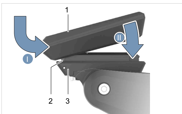
Figura 186: Montaggio del display
