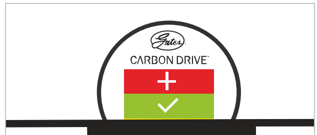
Figura 255: Esempio: indicatore sul bordo del settore giallo, per cui ridurre leggermente la tensione della cinghia
