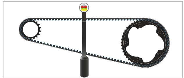
Figura 253: Asta di misura appesa
