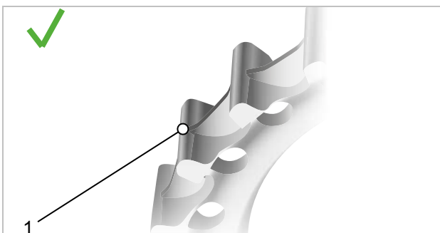
Figura 246: Profilo ottimale dei denti
