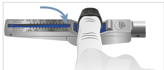
Figura 249: Dito indice nel calibro di verifica
