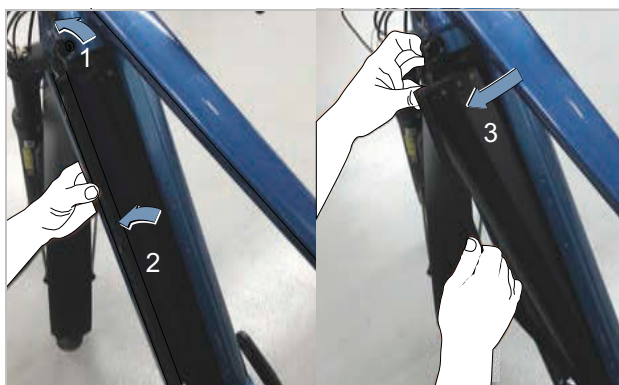
Figura 192: Montaggio della batteria integrata
