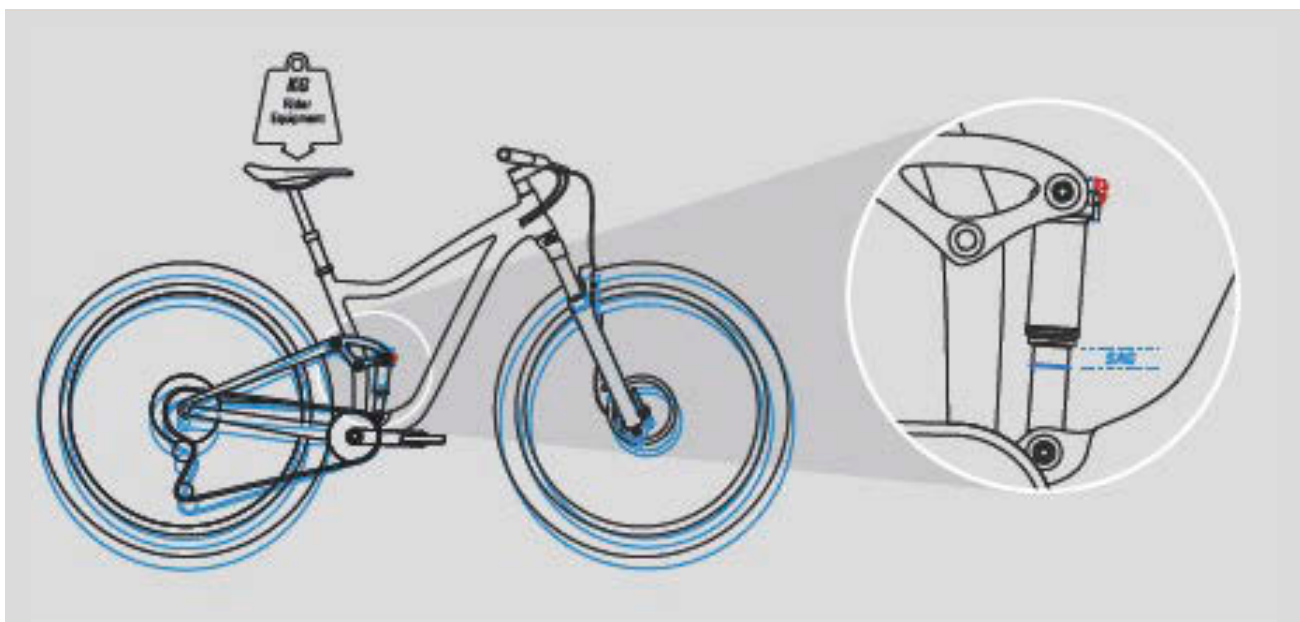
Figura 178: Ammortizzatore del carro posteriore SAG
