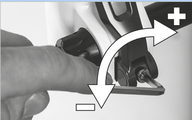
Figura 136: Regolazione della forza di serraggio del bloccaggio rapido
