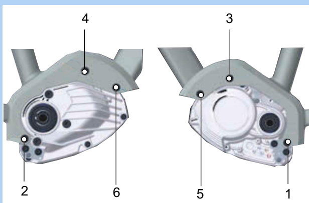
Figura 113: Ubicazione delle viti di fissaggio del motore da 1 a 6
