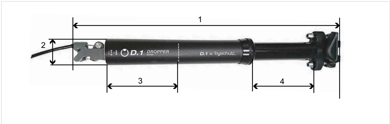
Figura 92: Dimensioni canotto reggisella BY,SCHUZ, D.1
