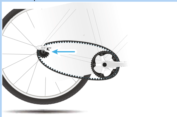
Figura 123: Spingere la ruota posteriore verso dietro
