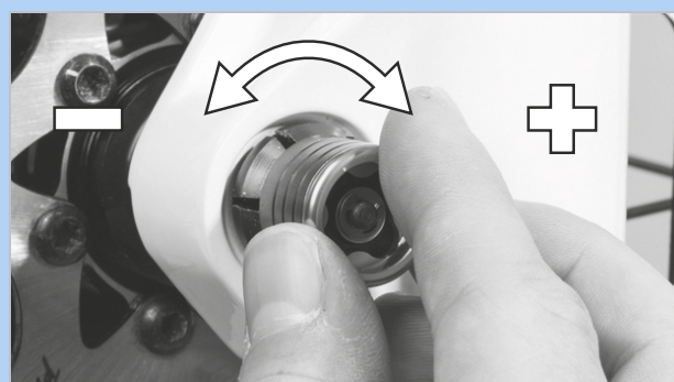
Figura 139: Regolazione del serraggio
