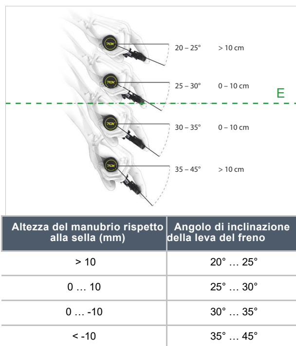
Figura 171: Angolo di inclinazione della leva del freno
