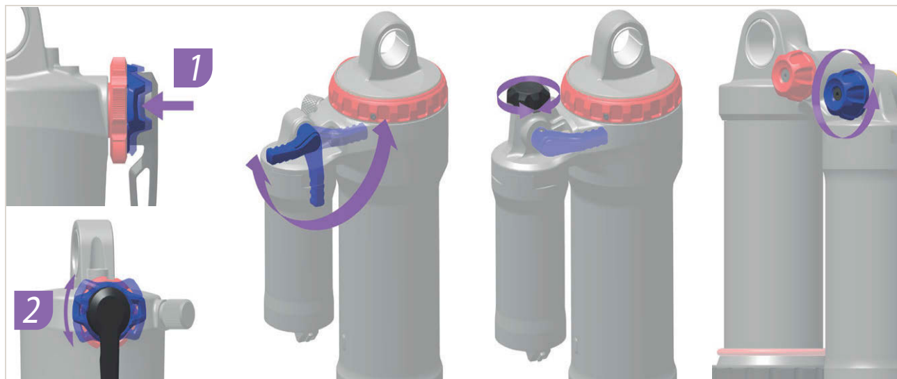
Figura 199: Ubicazione e forma dei regolatori dello stadio di compressione ROCKSHOX in diversi modelli
