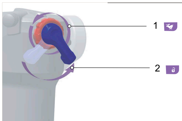
Figura 179: Apertura dell'ammortizzatore a stadi di trazione (1) e di pressione (2)
