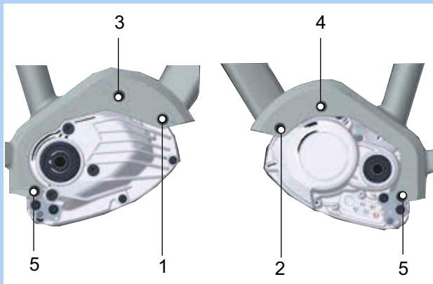
Figura 117: Ubicazione delle viti di fissaggio del motore da 1 a 6
