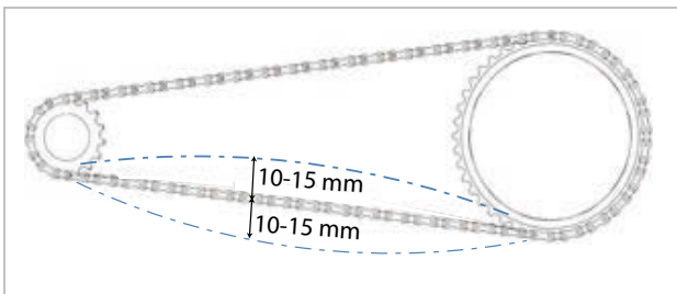
Figura 235: Controllo della tensione della catena, esempio: 5 mm verso l'alto, 10 mm verso il basso = scostamento 15 mm
