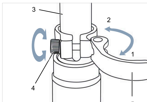
Figura 154: Apertura del bloccaggio rapido del canotto reggisella
