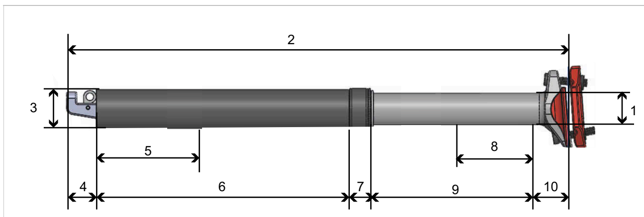
Figura 91: Dimensioni cannotto reggisella LIMOTEC, A3/A3 Plus
