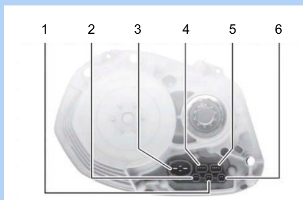
Slika 118: Položaj priključka motora Performance Line CX (BDU450 CX)
