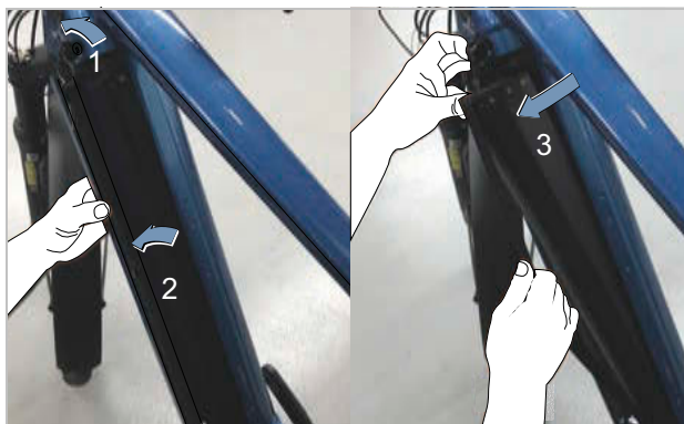
Slika 192: Umetanje integrirane baterije
