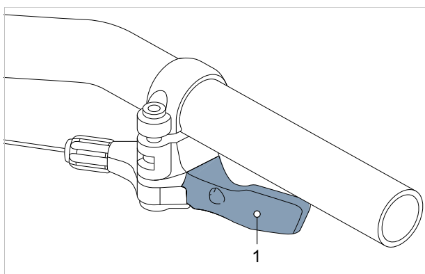
Slika 205: Upravljačka ručica daljinskog upravljača (1)
