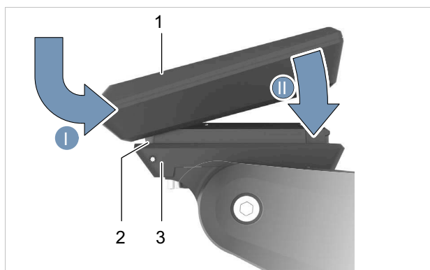
Slika 186: Umetanje zaslona
