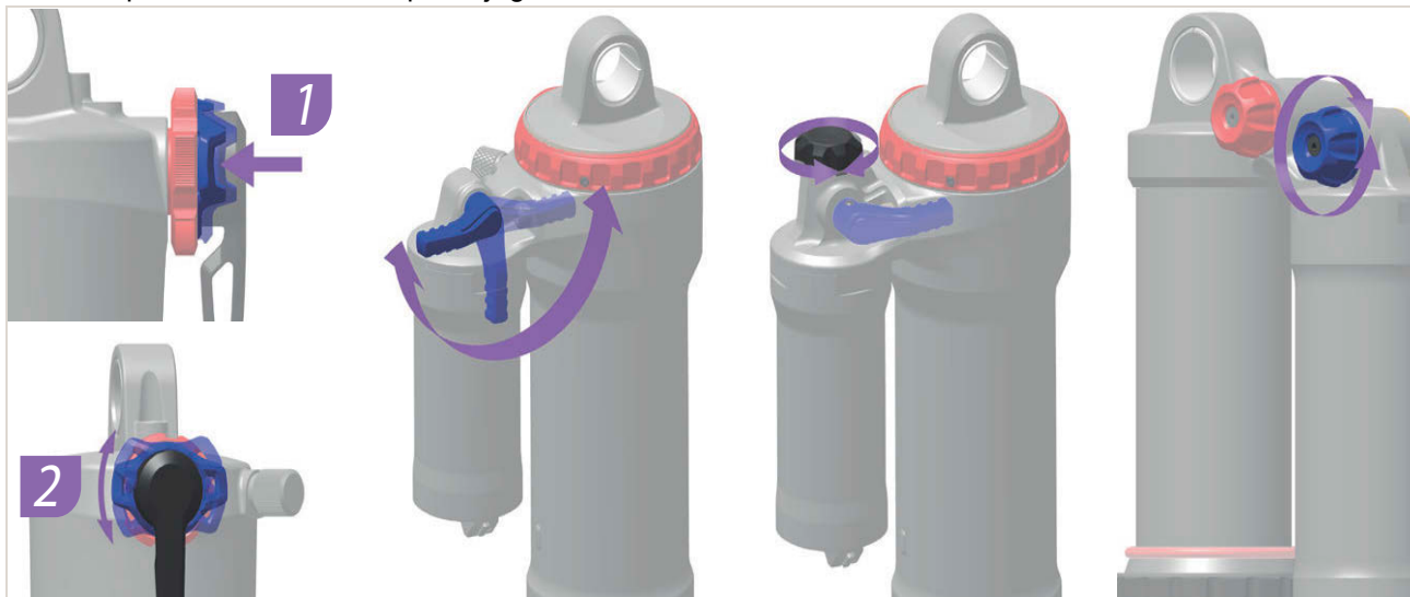
Slika 199: Položaj i oblik kotačića za podešavanje kompresije ROCKSHOX kod različitih modela
