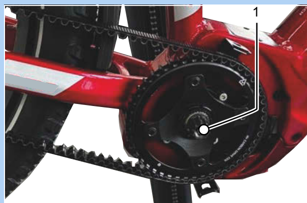
Slika 109: Otpuštanje remenice
