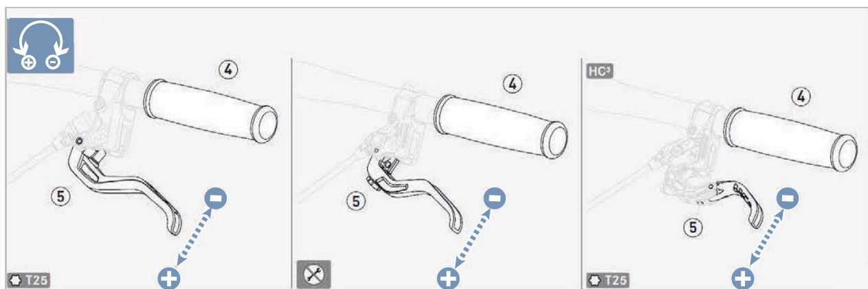
Slika 173: Podešavanje udaljenosti ručice kod MAGURA disk-kočnice
