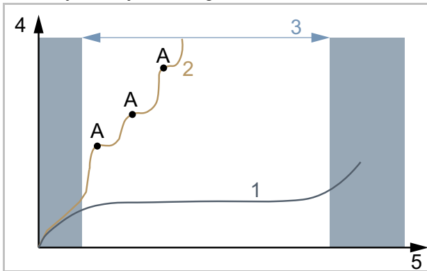
Slika 228: Grafikon trošenja: radni vijek (5) u odnosu na habanje materijala (4)
