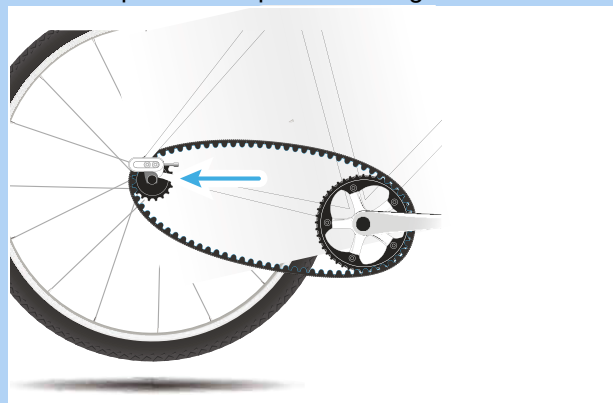
Slika 123: Pomicanje stražnjeg kotača prema natrag
