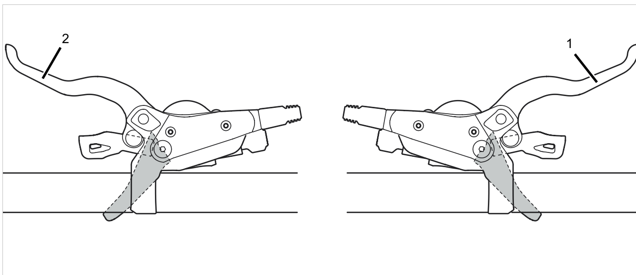
Slika 77: Ručna kočnica stražnjeg kotača (1) i prednjeg kotača (2), primjer kočnice SHIMANO
