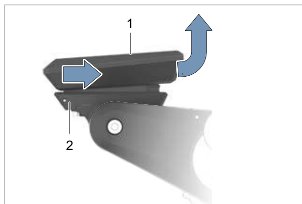
Slika 188: Skidanje biciklističkog računala
