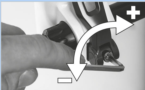
Slika 136: Podešavanje sile stezanja brzog zatvarača
