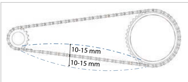
Slika 235: Primjer provjere zategnutosti lanca: 5 mm prema gore, 10 mm prema dolje = odstupanje od 15 mm
