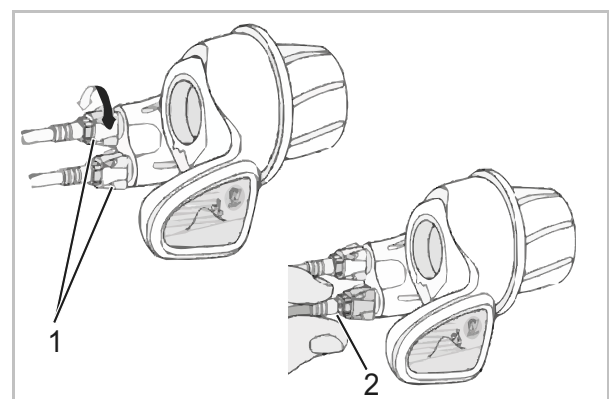
Slika 261: Okretnu ručicu mjenjača s čahurom za podešavanje (1) i rotacijskim zazorom (2)
