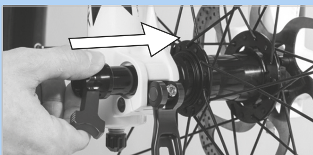
Slika 131: Uvlačenje poprečne osovine u smjeru strelice
