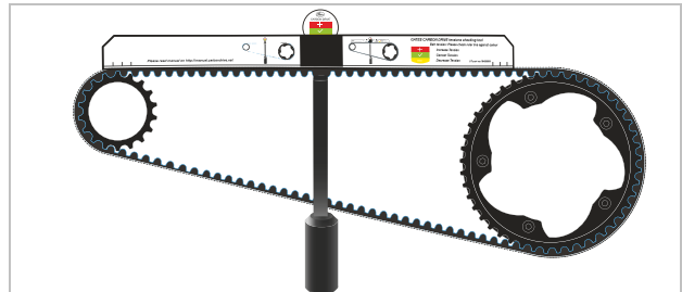
Slika 254: Postavljeno ravnalo
