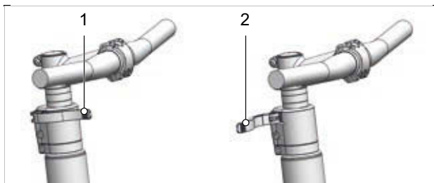
Slika 160: Zatvorena (1) i otvorena (2) stezna poluga lule, primjer All Up
