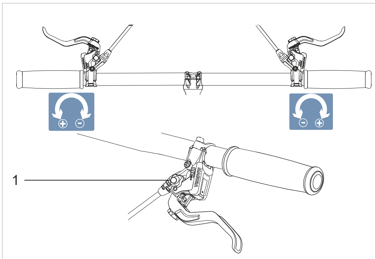
Slika 174: Uporaba okretnog gumba (1) za podešavanje pritisne točke
