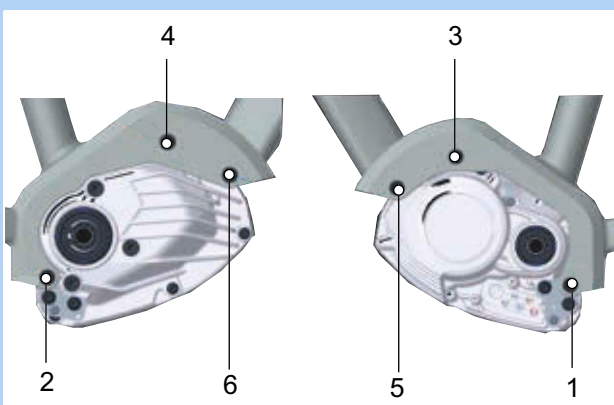
Slika 113: Položaj vijaka motora od 1 do 6
