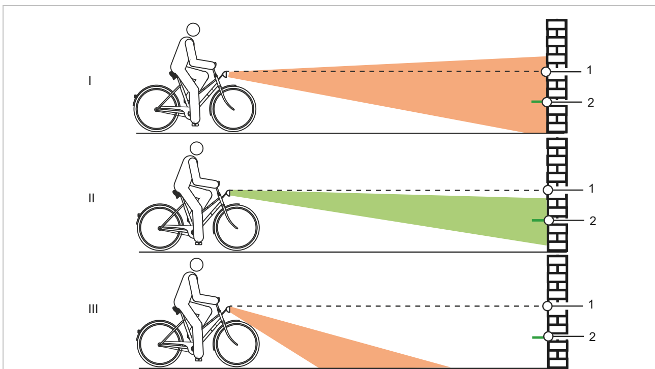
Slika 185: Svjetlo podešeno previsoko (1), ispravno (2) i prenisko (3)
