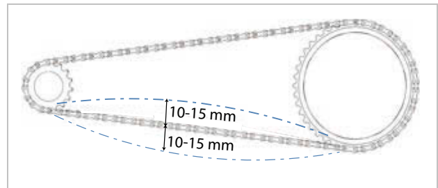
Slika 257: Primjer provjere zategnutosti lanca: 5 mm prema gore, 10 mm prema dolje = odstupanje od 15 mm
