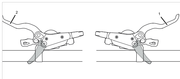
Slika 214: Ručna kočnica stražnjeg (1) i prednjeg kotača (2), primjer kočnice SHIMANO
