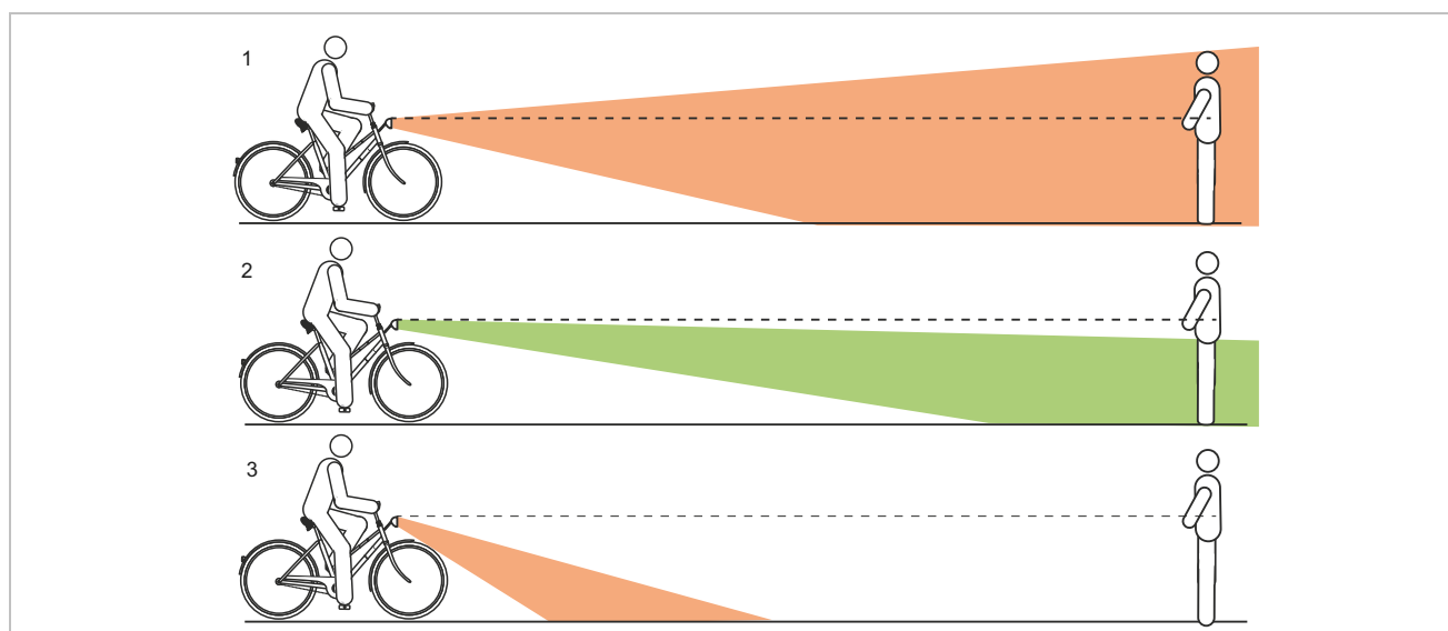
Slika 183: Svjetlo podešeno previsoko (1), ispravno (2) i prenisko (3)
