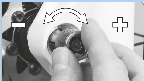
Slika 139: Podešavanje zategnutosti
