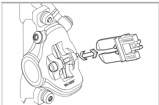
Slika 103: Pričvršćivanje zaštite za transport
