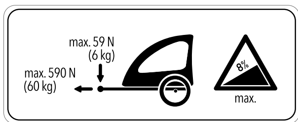
Slika 190: Napomena o prikolici
