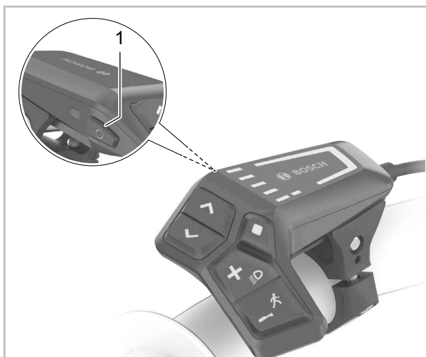
Slika 208: Položaj tipke za uključivanje i isključivanje na uređaju BOSCH LED Remote
