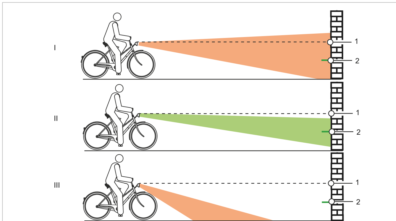
Illustration 180 : Feu réglé trop haut (1), correctement (2) et trop bas (3)
