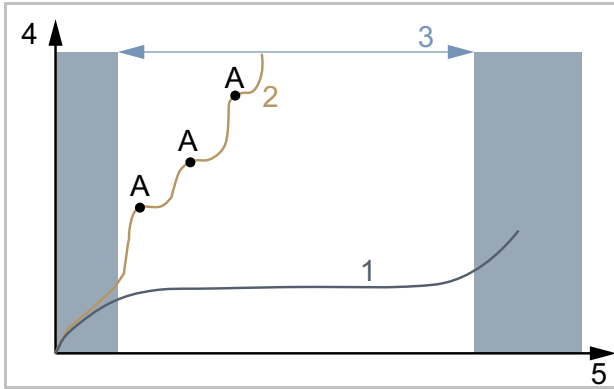
Illustration 162 : Diagramme d'usure, durée de service (5) par rapport à l'enlèvement de matière (4)
