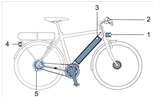
Illustration 47 : Schéma du système d'entraînement électrique avec composants électriques
