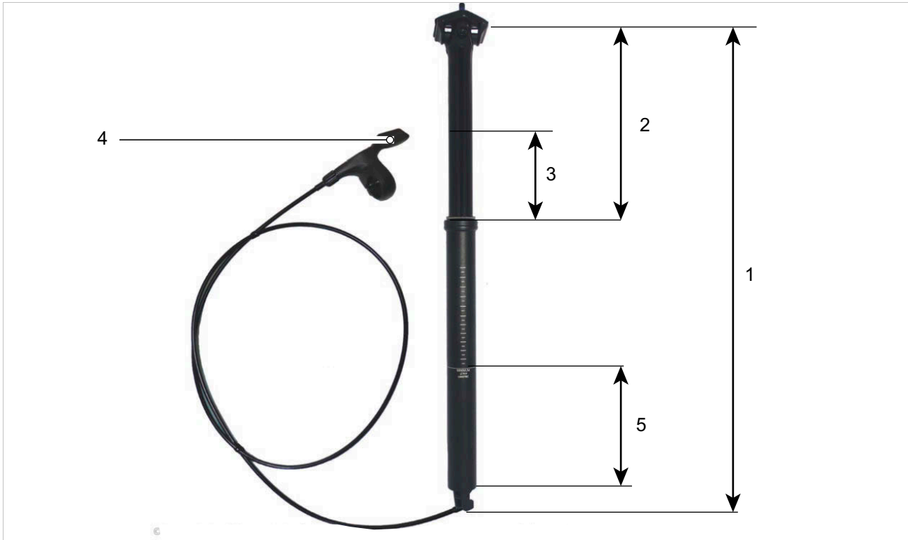
Illustration 43 : Structure et dimensions de la tige de selle LIMOTEC A3
