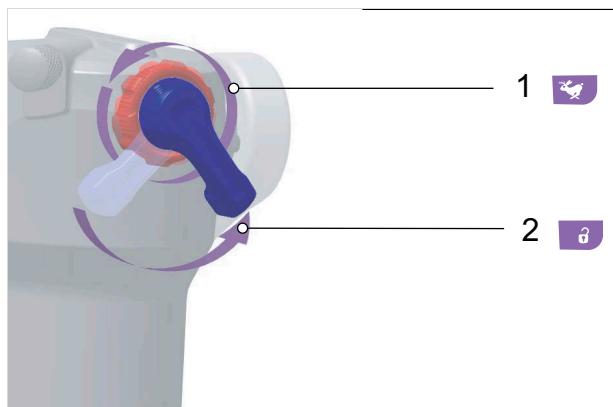
Illustration 121 : Ouvrir l'amortisseur de détente (1) et l'amortisseur de compression (2)
