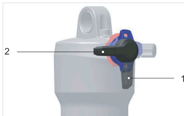
Illustration 147 : Position ouverte (1) et position du seuil (2) sur l'amortisseur arrière (noir)
