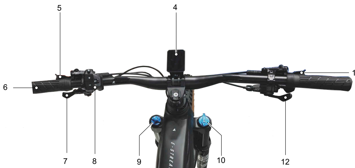
Illustration 52 : Vue détaillée du guidon avec ordinateur de bord FIT Remote Basic et écran Compact 2.0, exemple
