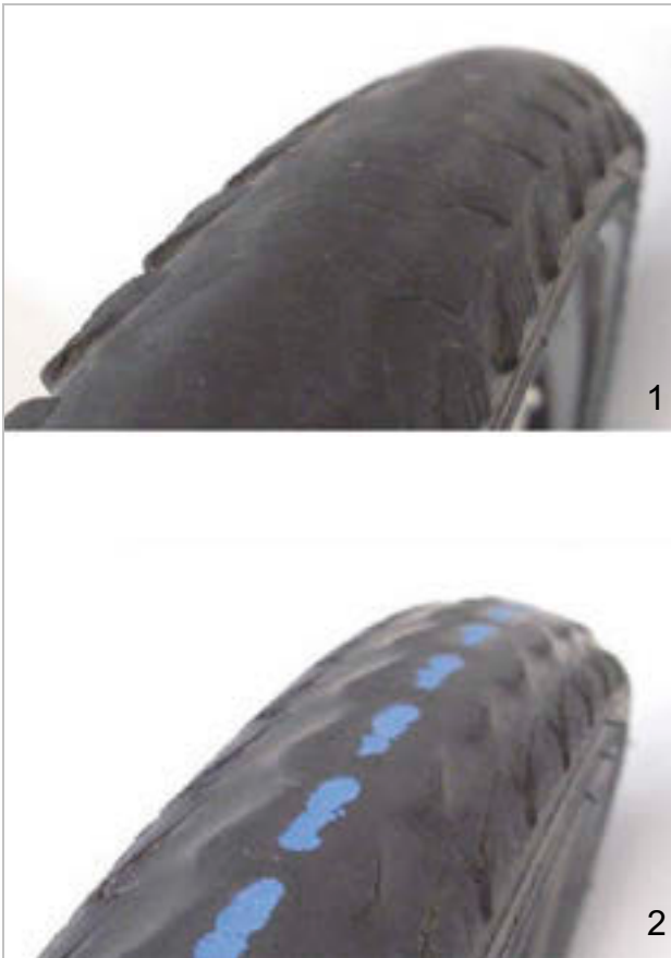
Illustration 166 : Pneu sans profil pouvant être changé (1) et pneu avec protection anti-crevaison visible (2) devant être changé
