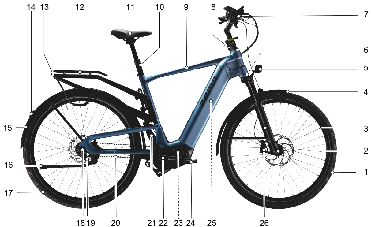
Illustration 3 : Vélo électrique vu de droite, exemple
